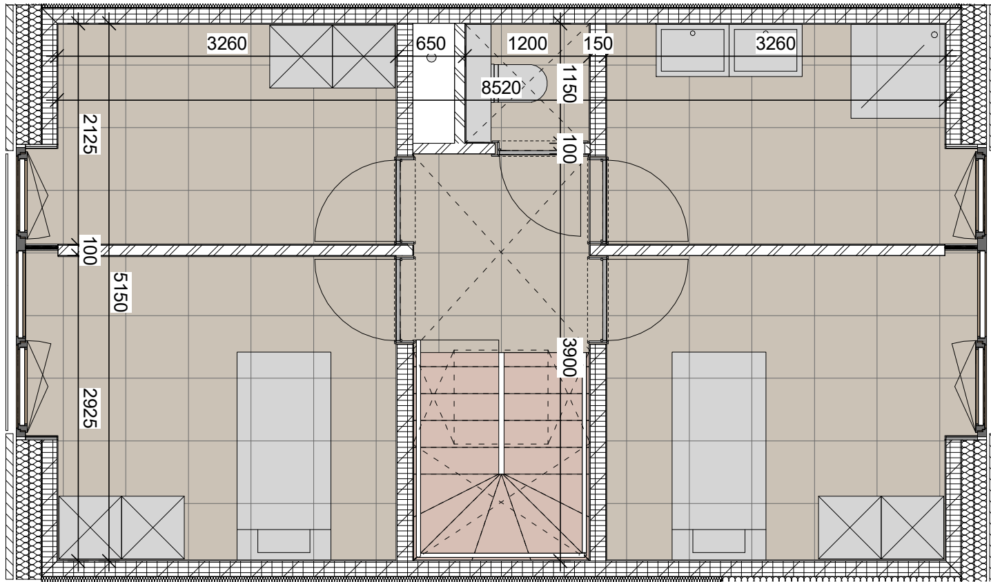
2de verdieping
